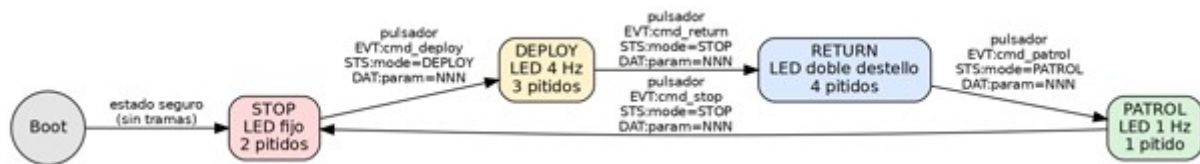
Figura 4 — Diagrama de estados de la caja de comandos con las tramas emitidas en cada transición.
