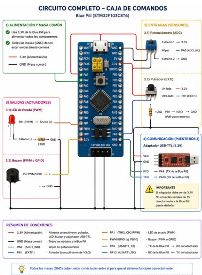
Figura 1 — Esquema de conexión del puesto. GND común entre todos los componentes.
