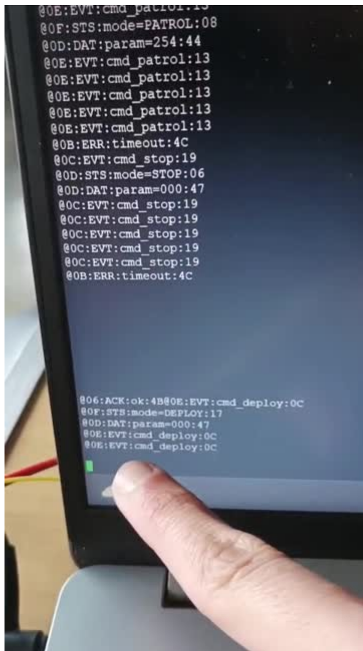
Figura 8 — Fotograma de la prueba UART: ACK:ok confirma la recepción del evento.
