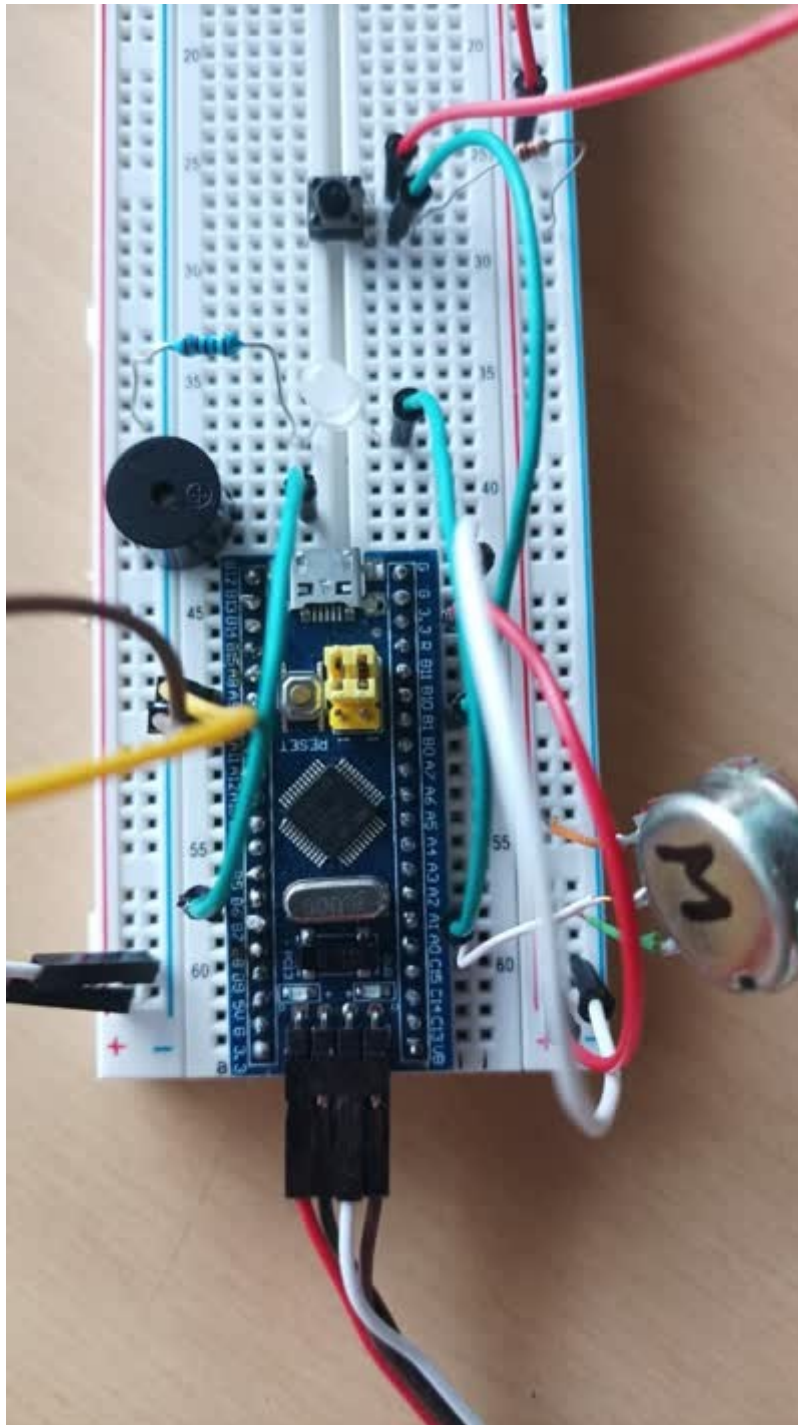
Figura 6 — Montaje físico de la caja de comandos: Blue Pill, pulsador, LED, buzzer y potenciómetro.
